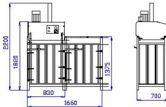
Dvoukomorový lis EKOPACK 100.2
