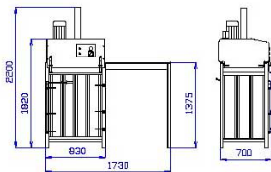
Jednokomorový lis EKOPACK 100.1
